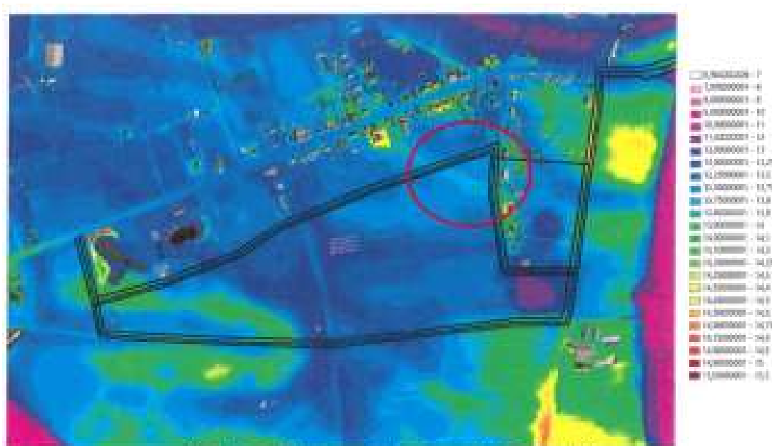
Afbeelding 5: Hoogteverschil deelgebied Ven-Zelderheide (bron: presentatie overleg T2G en project Lob van Gennep (19-03-2021))
