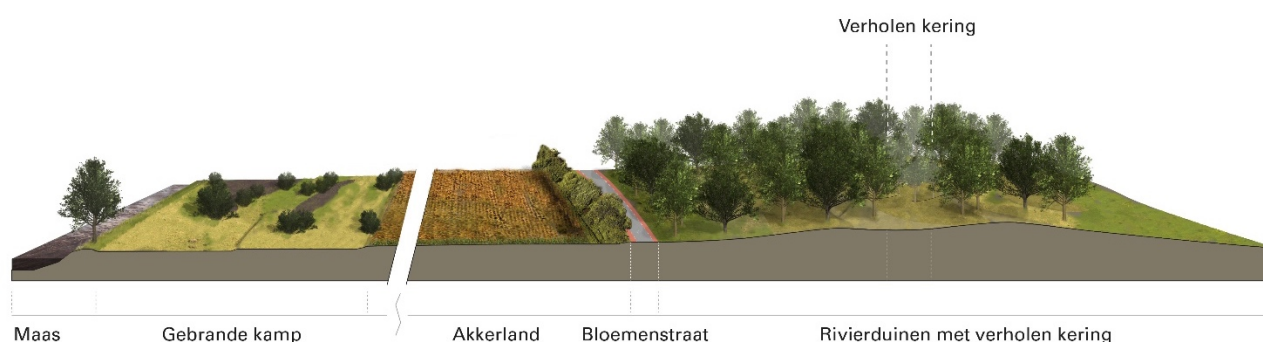
Afbeelding 20: Perspectiefdoorsnede verborgen waterkering gecombineerd met rivierduinen
