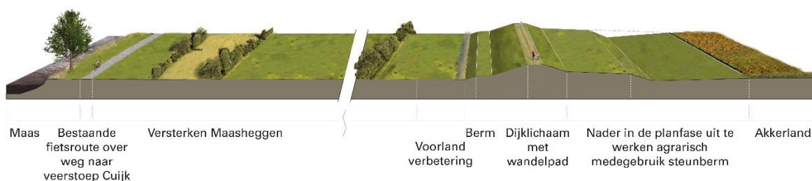
Afbeelding 13: Perspectief doorsnede dijkversterking deelgebied Maasdal
