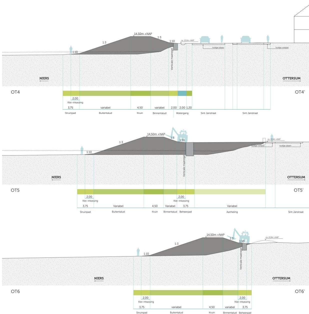
Figuur 2.4: Dwarsprofielen dijktracé sportvelden Achates
