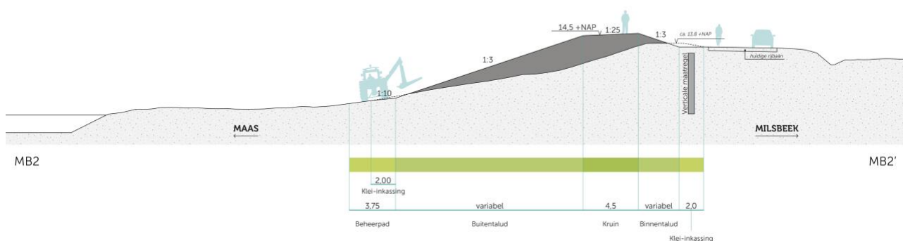
Figuur 2.4: Dwarsprofiel dijktracé Bloemenstraat vanaf rijksweg N271
