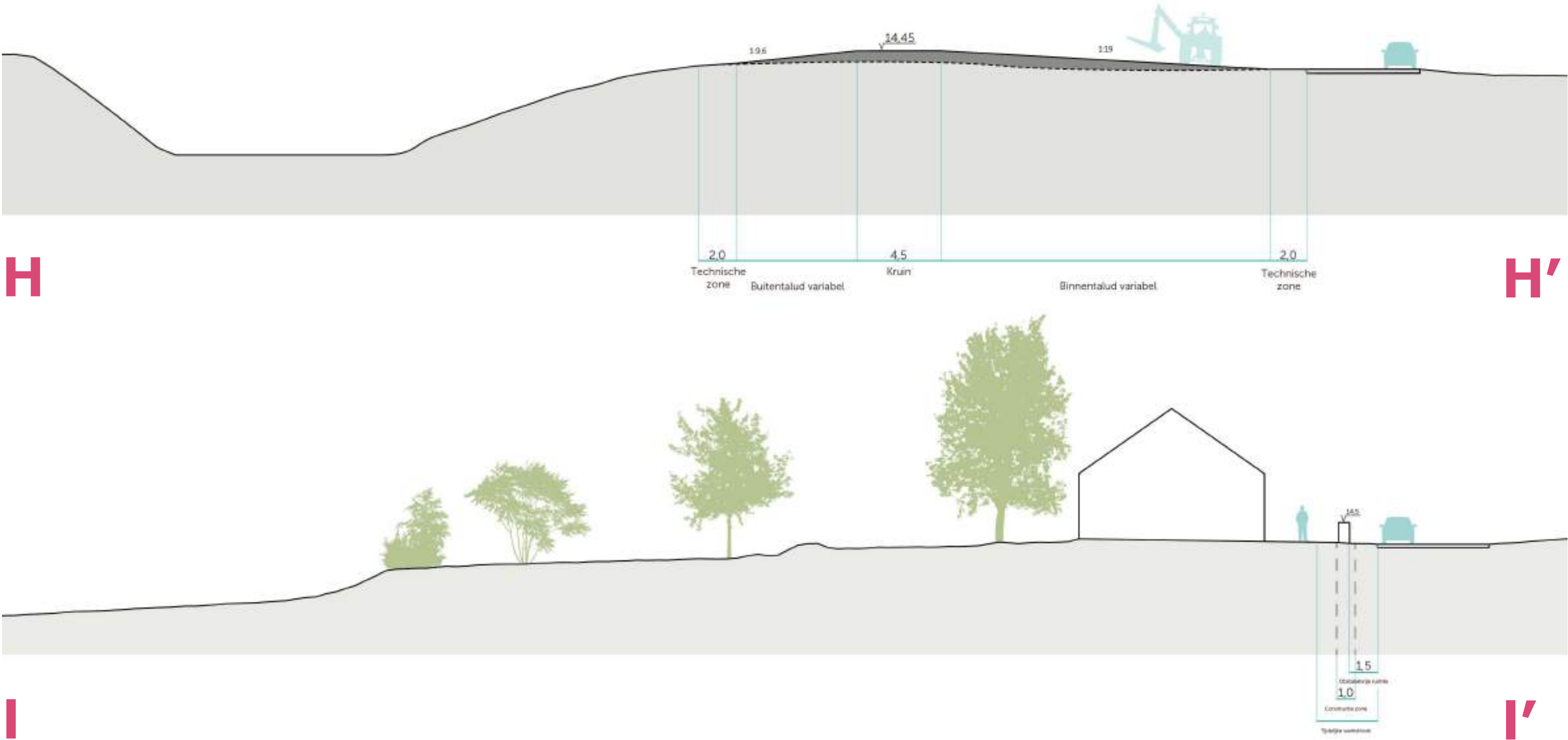
Profiel en maatvoering onder voorbehoud van verdere berekeningen en detaillering
