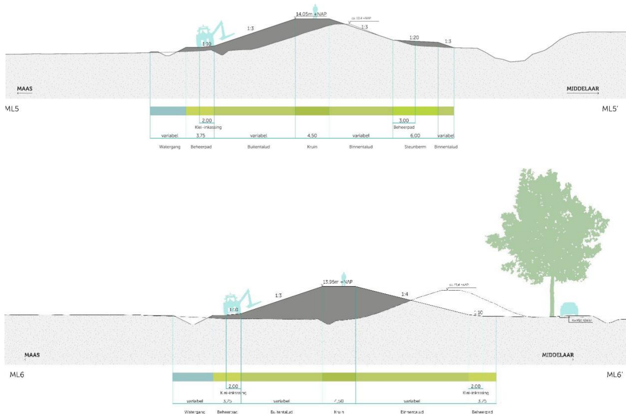
Figuur 2.2: Profielen dijktracé Kopsesweg – Fuikstraat
